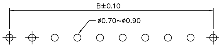
P.C.B. Layout
